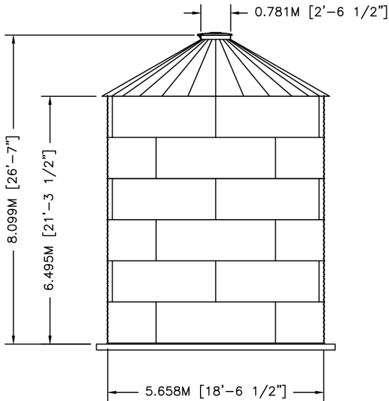
ELEVATION
